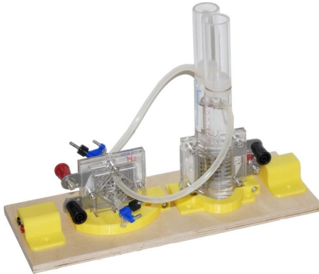
Elektrolyseur und Brennstoffzelle
